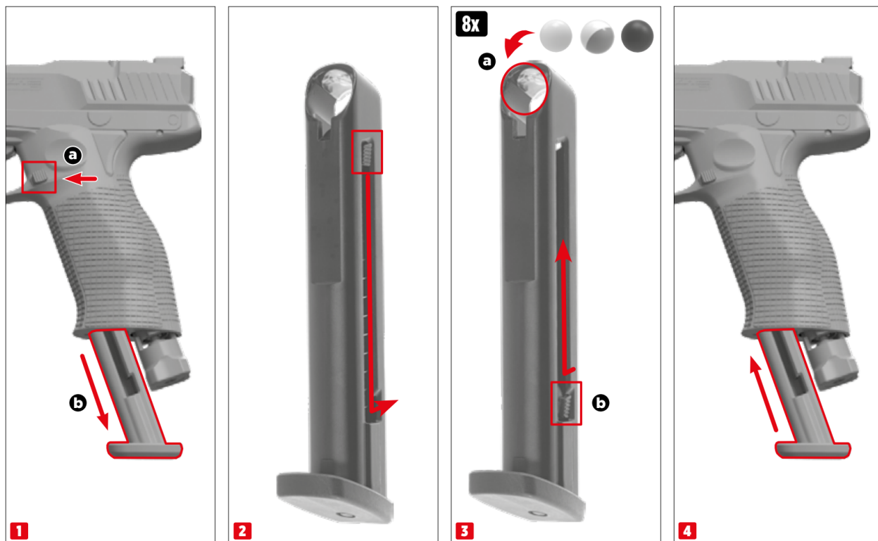
Vyjmutí (1), stažení pružiny (2), nabití (3) a zasunutí zásobníku (4)
