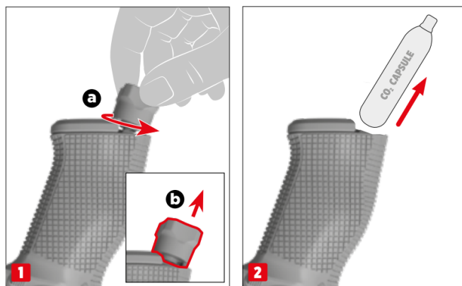
Vyjmutí uzávěru (a, b) a prázdné bombičky
