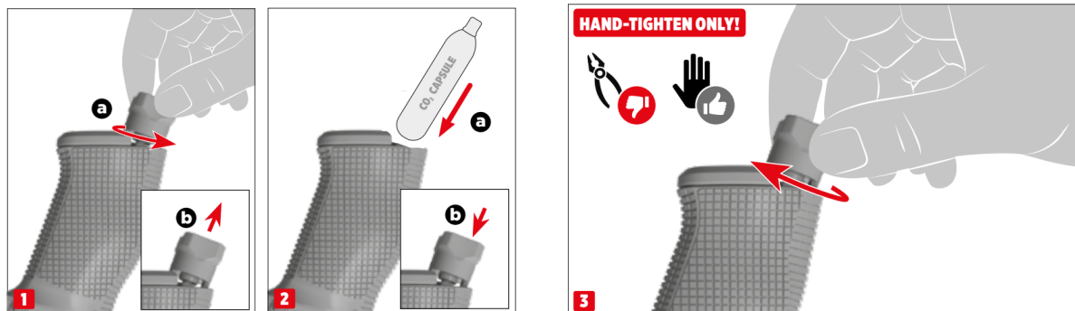
Krok 1–2: vyšroubování uzávěru (a, b) a vložení CO2 bombičky
